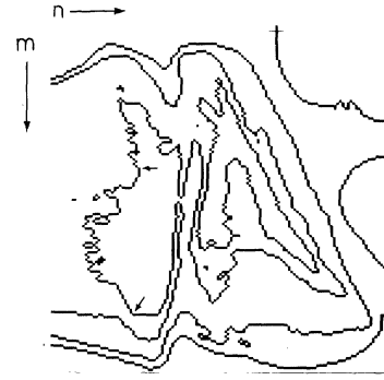
Fig. 4. Input image.
