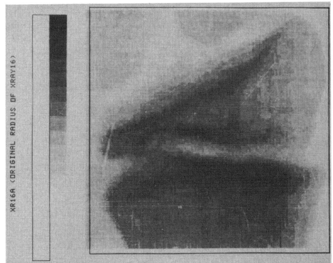
Fig. 5. Input image.
